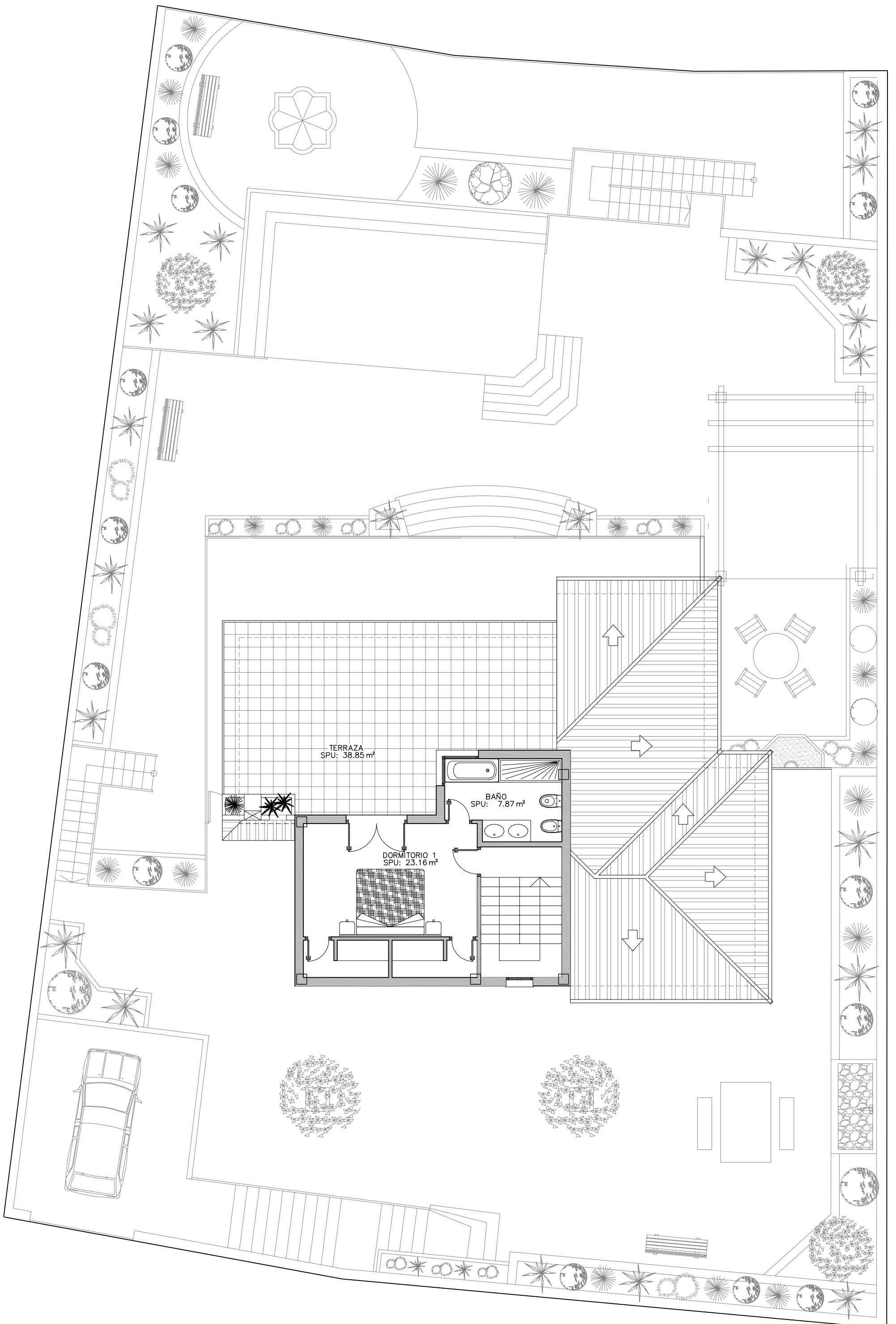
PLANTA DE CUBIERTA ESCALA 1/100
