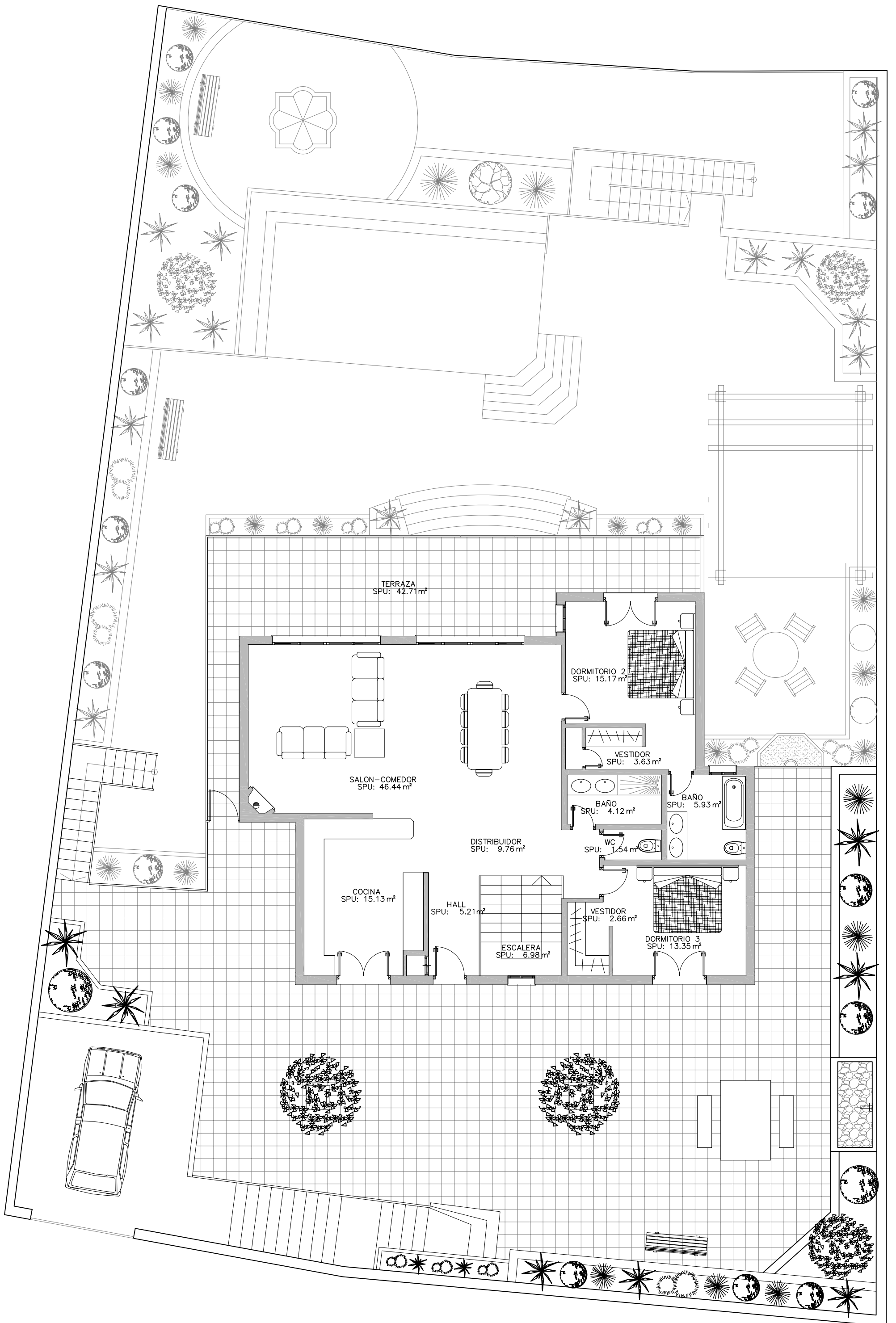
PLANTA BAJA Y ACCESO A PARCELA ESCALA 1/100
